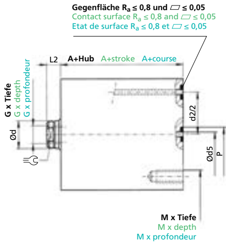
Bei Funktionsart 204 / 208 With operation mode 204 / 208 Pour le type de fonctionnement 201 / 206
